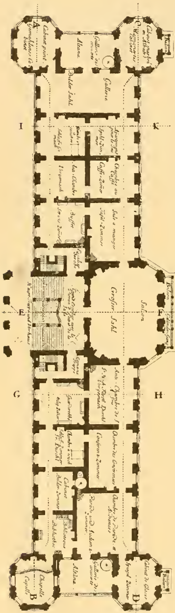
Fig. 67. Schloss Belvedere zu Wien. Hauptgeschoß.
